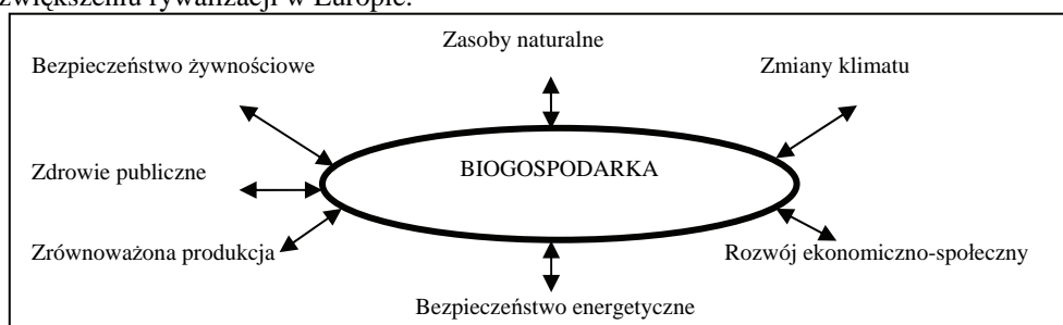
Rys. 1. Oddziaływanie biogospodarki
